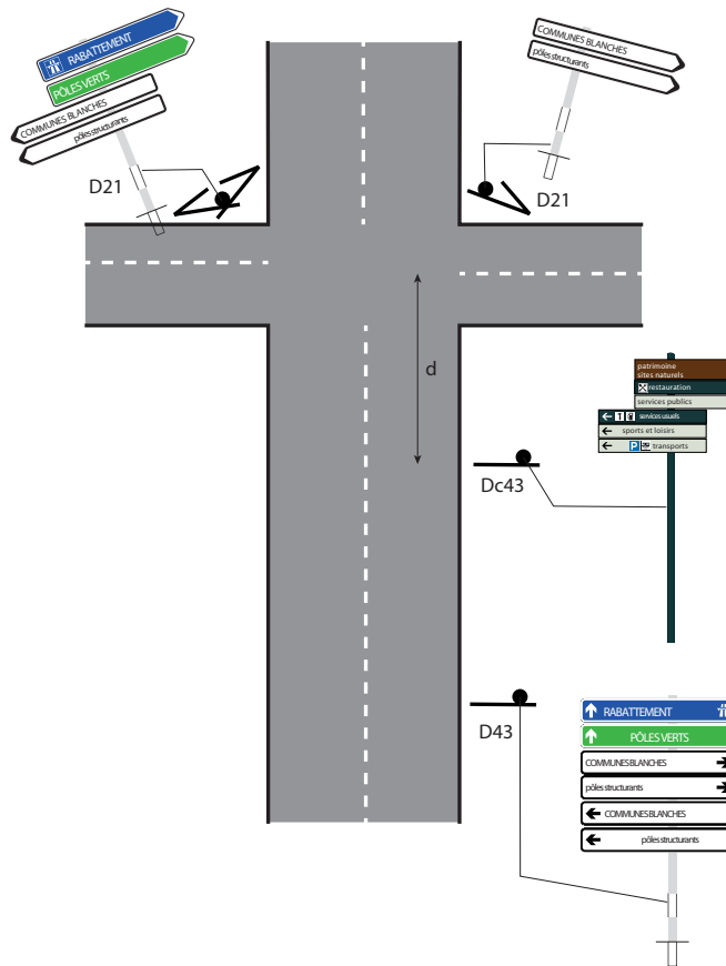
Carrefour équipé de signalisation directionnelle routière
